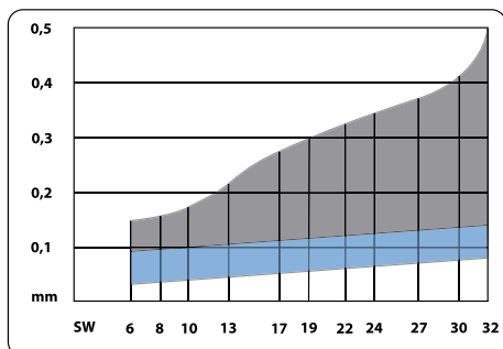
GEDORE DIN стандарт SW = размер ключа
