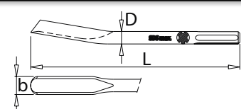
651.3 ЗУБИЛО КАНАВЧАТОЕ, ПОСАДКА SDS-МАКС
